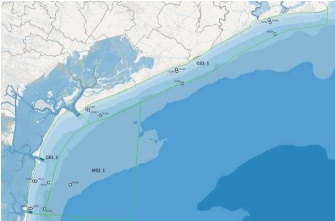
Figura 10.7: Localizzazione dei 5 transetti di monitoraggio ARPAV situati nel Compartimento Marittimo di Venezia.
