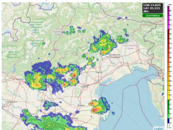
Figura 6 – Ore 15.00 legali: ripresa delle precipitazioni con rovesci e temporali sparsi
