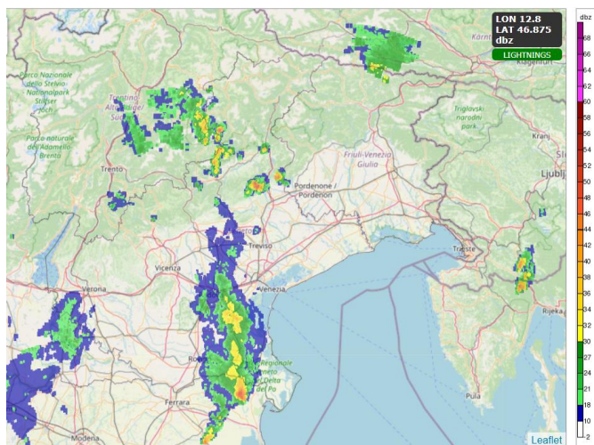
Figura 15 – Ore 14.00 legali: precipitazioni in ripresa nel pomeriggio, a carattere sparso.
