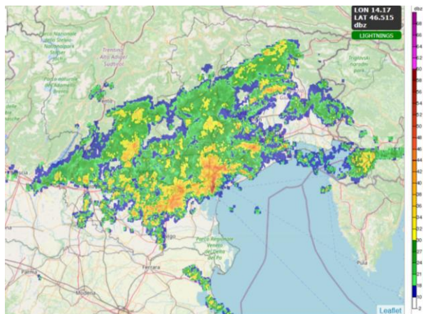
Figura 11 – Ore 06.30 legali: precipitazioni diffuse sui settori della pianura centro-settentrionale e orientale, con rovesci e temporali. Si noti la persistenza di rovesci tra le province di Padova e Venezia.
