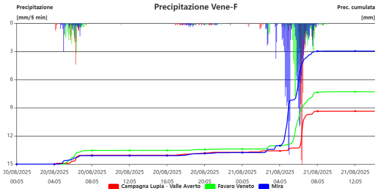
Figura 17 – Ietogramma delle stazioni maggiormente interessate dall'evento nella zona Vene-F
