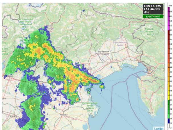
Figura 4 – Ore 06.00 legali: precipitazioni diffuse, con rovesci e temporali su settori centro-occidentali
