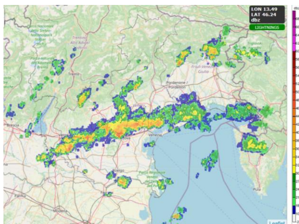
Figura 9 – Ore 04.00 legali: linea di precipitazioni con rovesci e temporali sulla pianura
