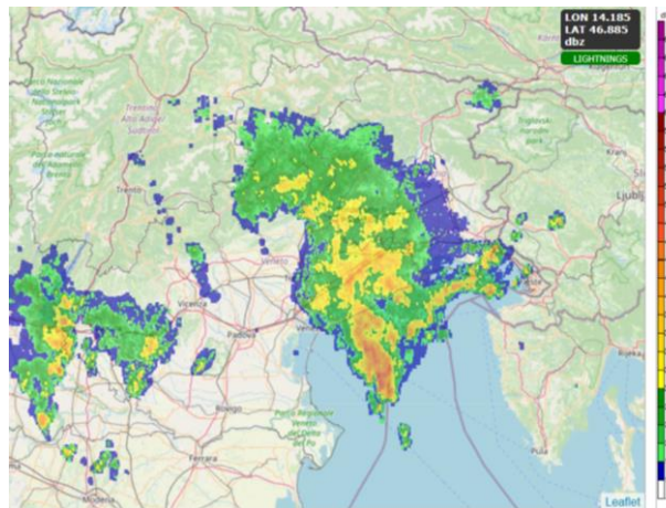
Figura 14 – ore 10.00 legali: precipitazioni diffuse sui settori della pianura settentrionale e orientale, con rovesci e temporali. Si noti la persistenza di rovesci tra le province di Venezia.
