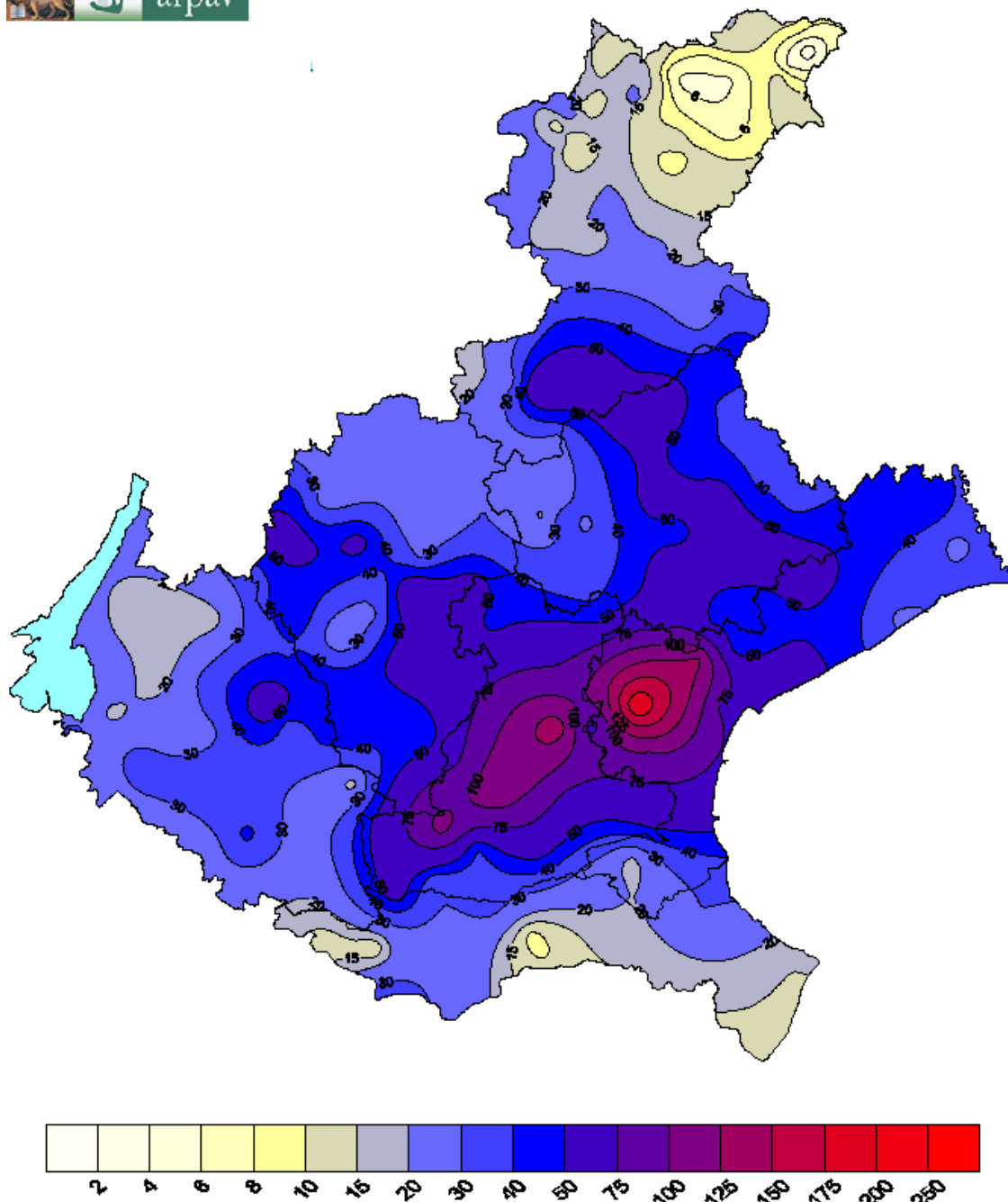
Figura 3 – Mappa con le precipitazioni cumulate delle due giornate di mercoledì 20 e giovedì 21 agosto 2025 [mm/24h].
