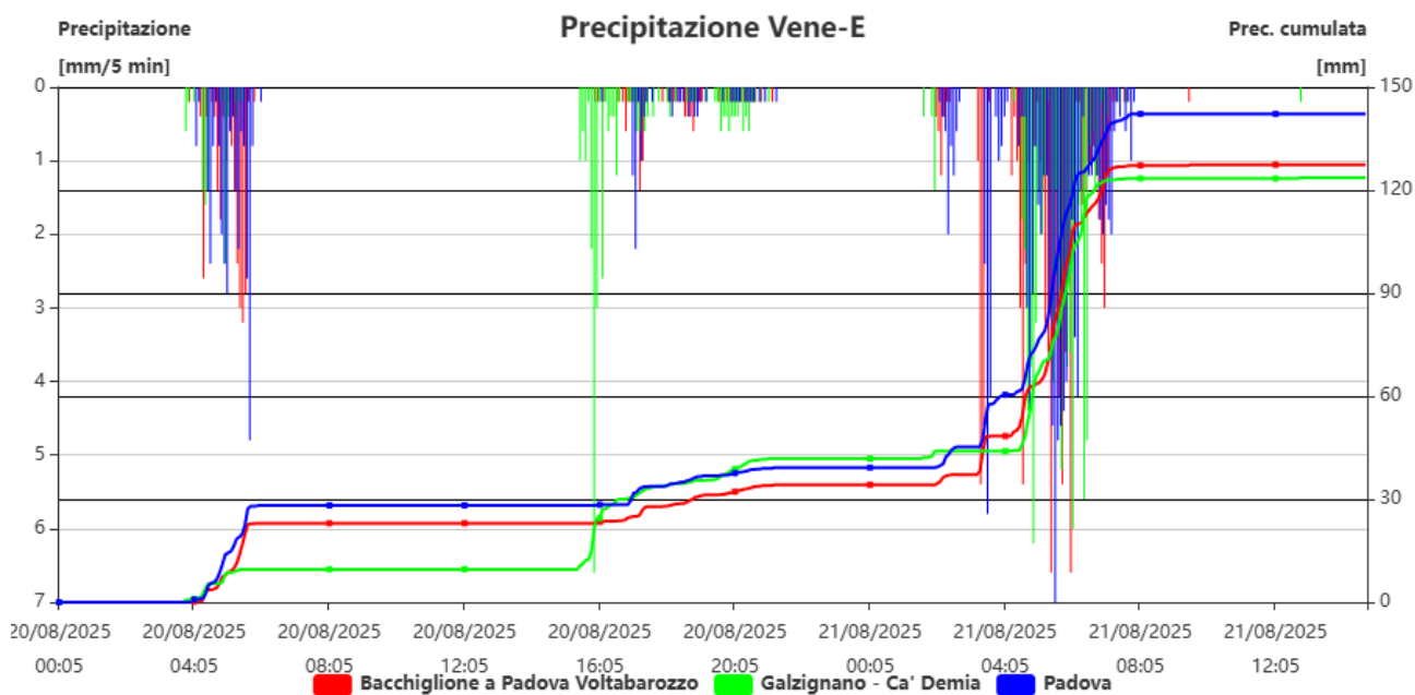
Figura 16 – Ietogramma delle stazioni maggiormente interessate dall'evento nella zona Vene-E
