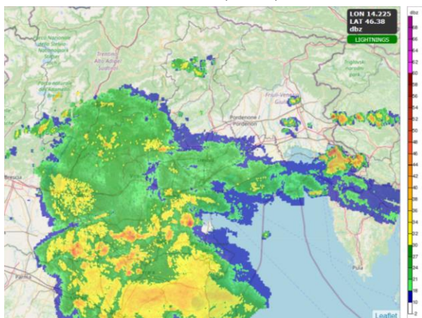
Figura 8 – Ore 20.00 legali: precipitazioni diffuse sulla pianura
