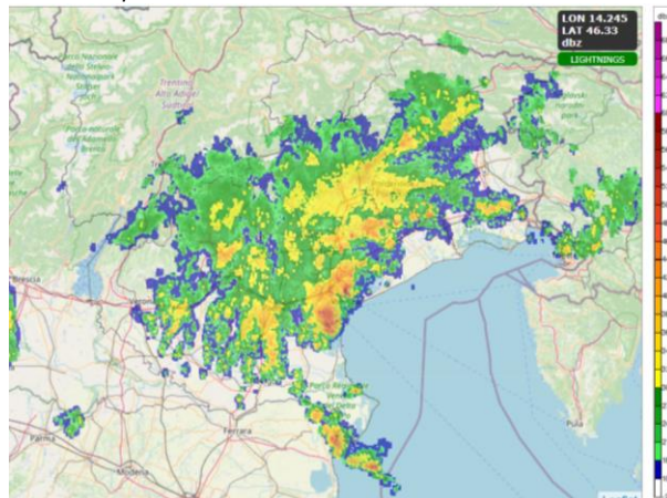
Figura 12 – Ore 07.30 legali: precipitazioni diffuse sui settori della pianura centro-settentrionale e orientale, con rovesci e temporali. Si noti la persistenza di rovesci tra le province di Padova e Venezia.
