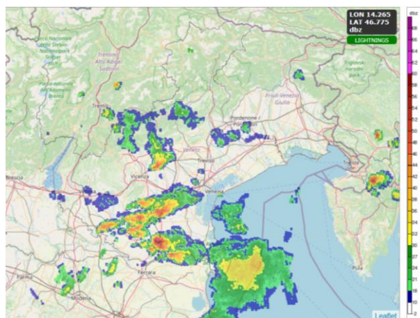
Figura 7 – Ore 17.00 legali: ripresa delle precipitazioni con rovesci e temporali sparsi
