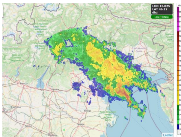
Figura 5 – Ore 08.00 legali: precipitazioni diffuse, in spostamento verso nord-est
