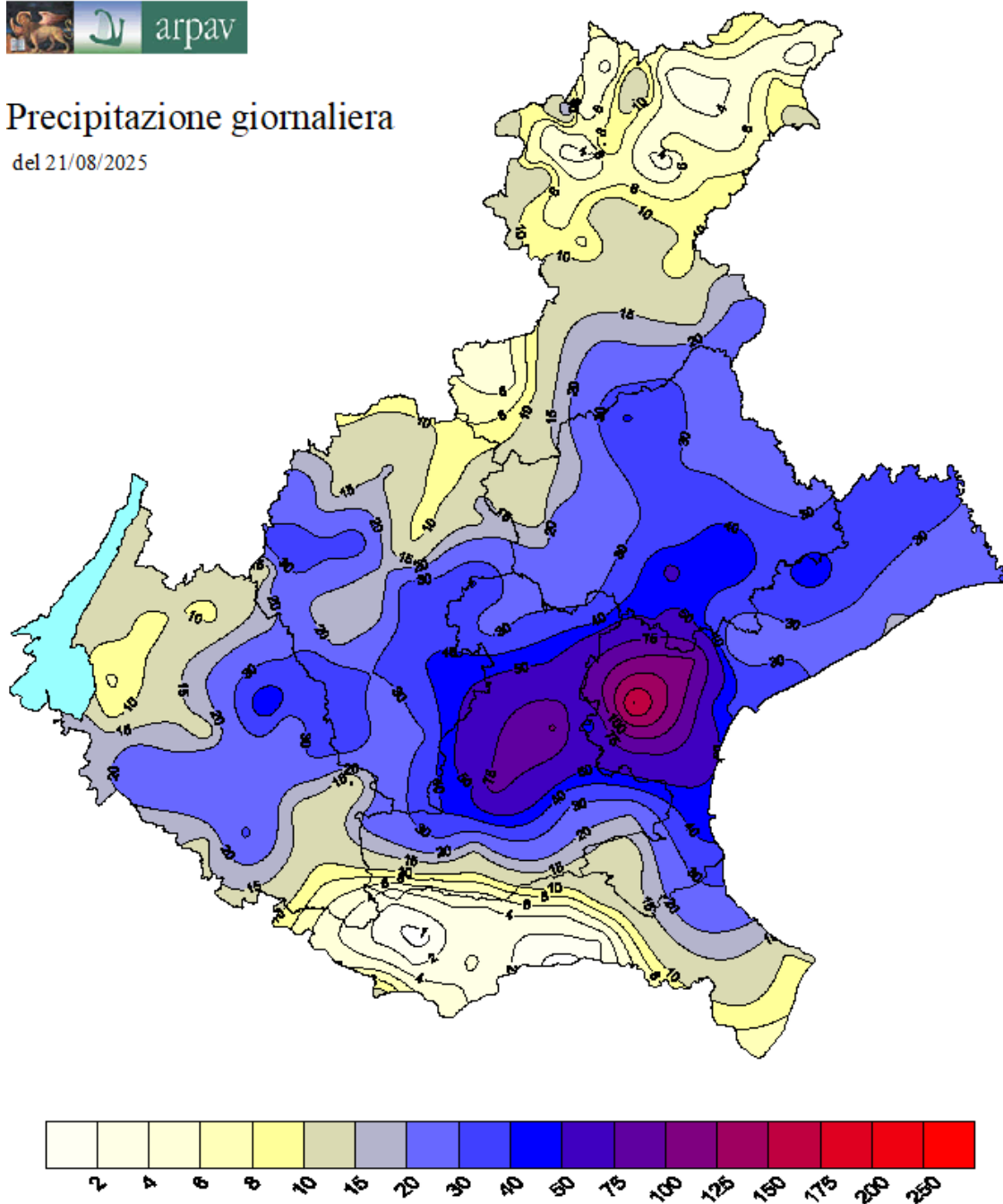
Figura 2 – Mappa con le precipitazioni cumulate di giovedì 21 agosto 2025 [mm/24h].
