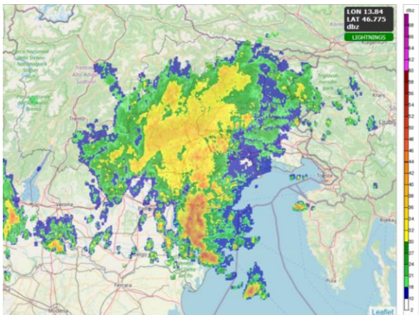
Figura 13 – ore 09.00 legali: precipitazioni diffuse sui settori della pianura settentrionale e orientale, con rovesci e temporali. Si noti la persistenza di rovesci tra le province di Venezia.
