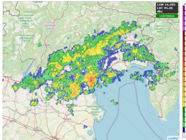
Figura 10 – 06.00 legali: precipitazioni diffuse sui settori della pianura centro-settentrionale e orientale, con rovesci e temporali. Si noti il nucleo intenso sul Veneziano.
