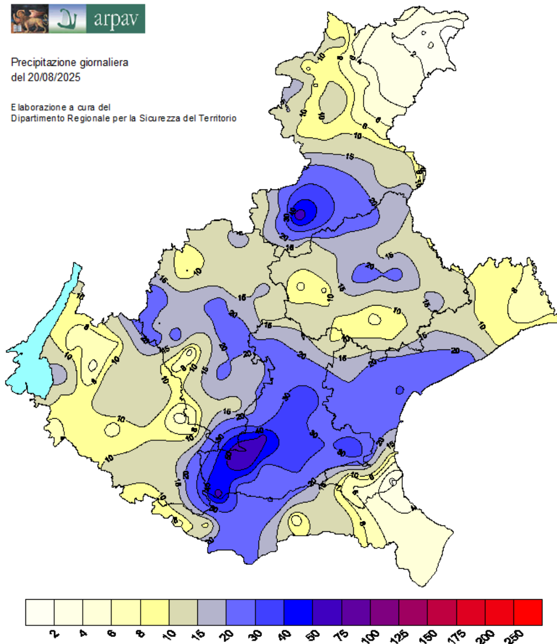
Figura 1 – Mappa con le precipitazioni cumulate di mercoledì 20 agosto 2025 [mm/24h].
