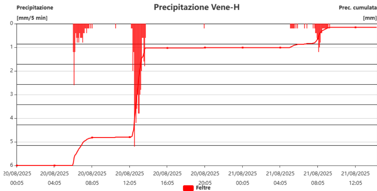
Figura 18 – Ietogramma delle stazioni maggiormente interessate dall'evento nella zona Vene-H
